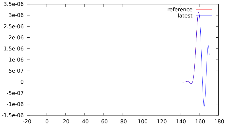
SR.BGIO.MXZ.sem.ascii
