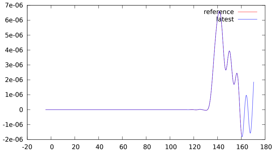
YL.BEKI.MXN.sem.ascii
