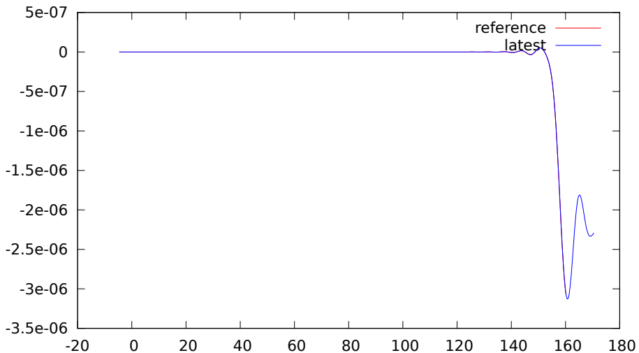
SR.BGIO.MXN.sem.ascii
