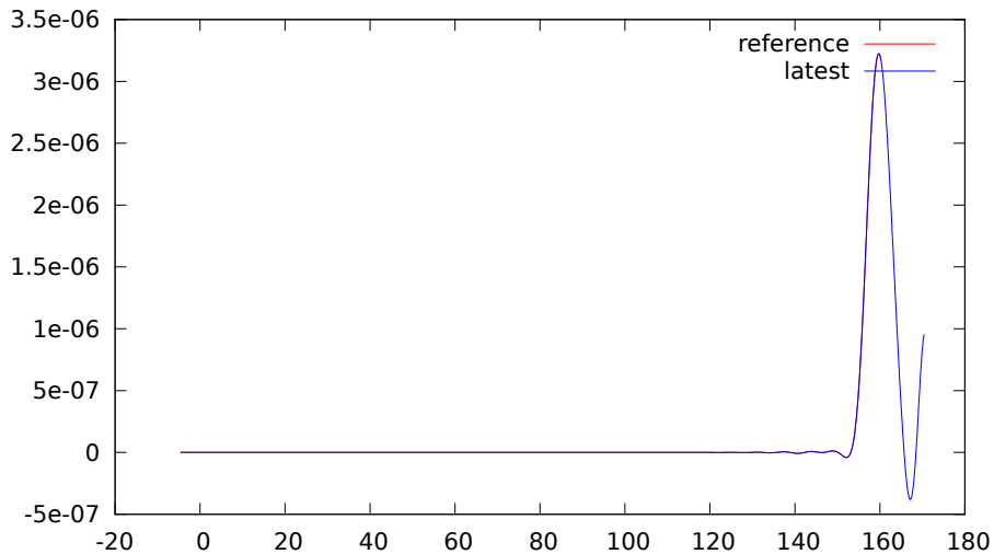
SR.BGIO.MXE.sem.ascii
