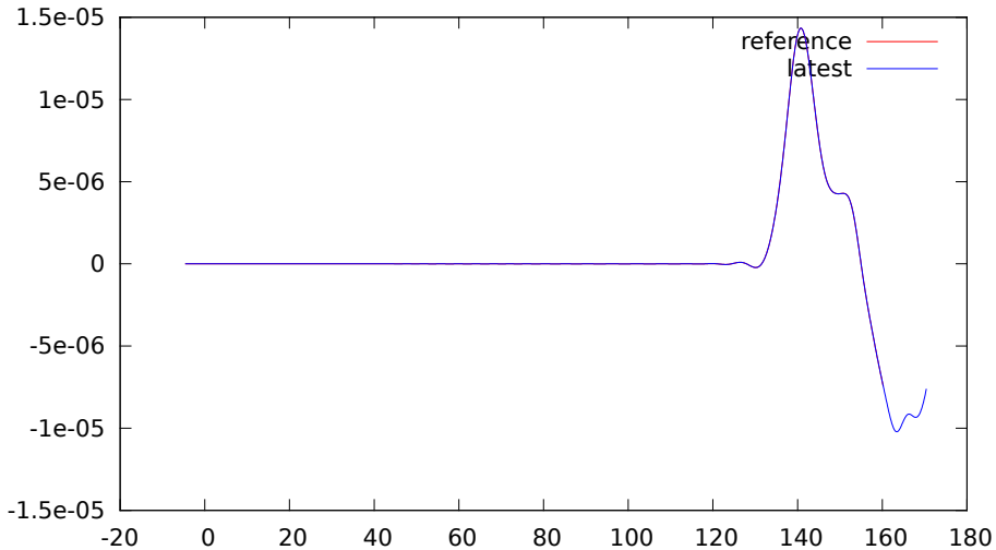
YL.BEKL.MXE.sem.ascii
