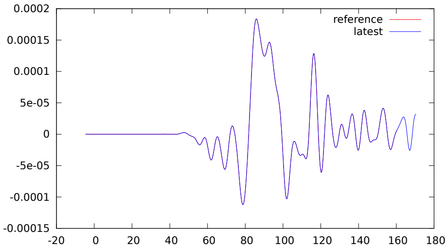
GE.ZKR.MXN.sem.ascii
