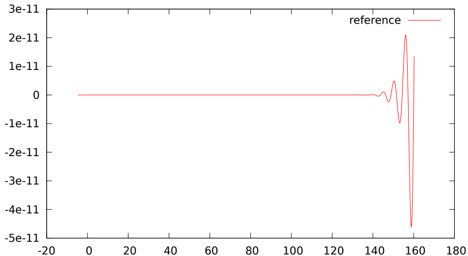
IU.GRFO.MXE.sem.ascii
