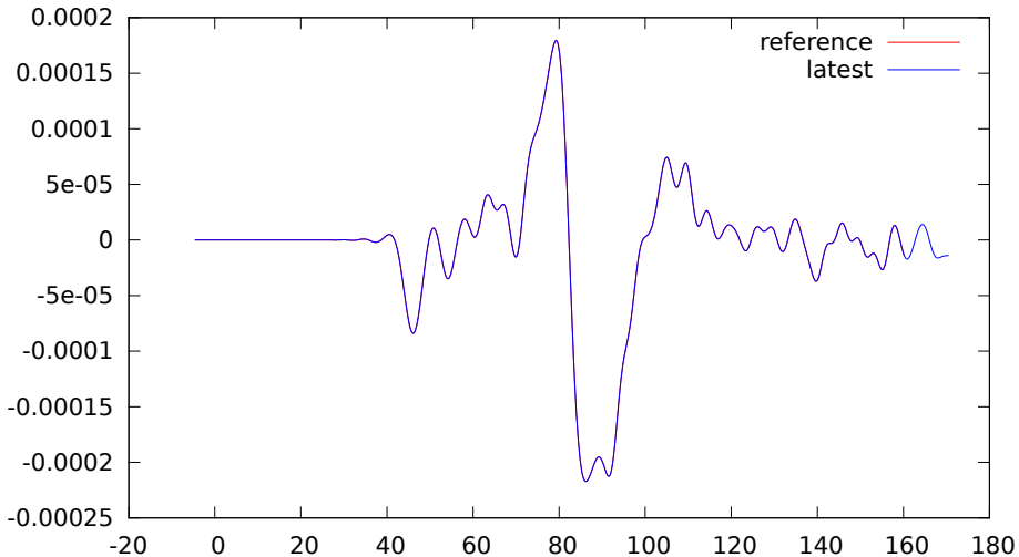
HT.LIT.MXZ.sem.ascii
