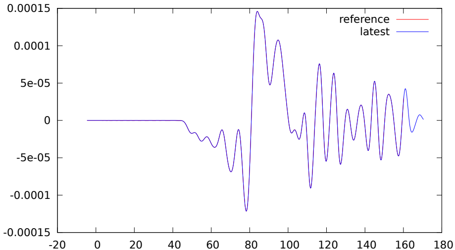
GE.ZKR.MXE.sem.ascii
