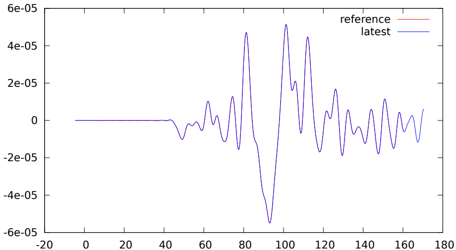
GE.ZKR.MXZ.sem.ascii
