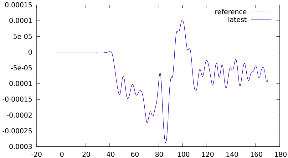
HT.LIT.MXN.sem.ascii
